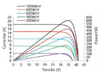
Curva de corrente/potência- tensão SS9-60HS-600M
