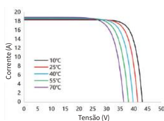
Curva de corrente e tensão SS9-60HS-600M
