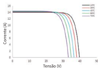
Curva de corrente e tensão SS8-54HDB-420N
